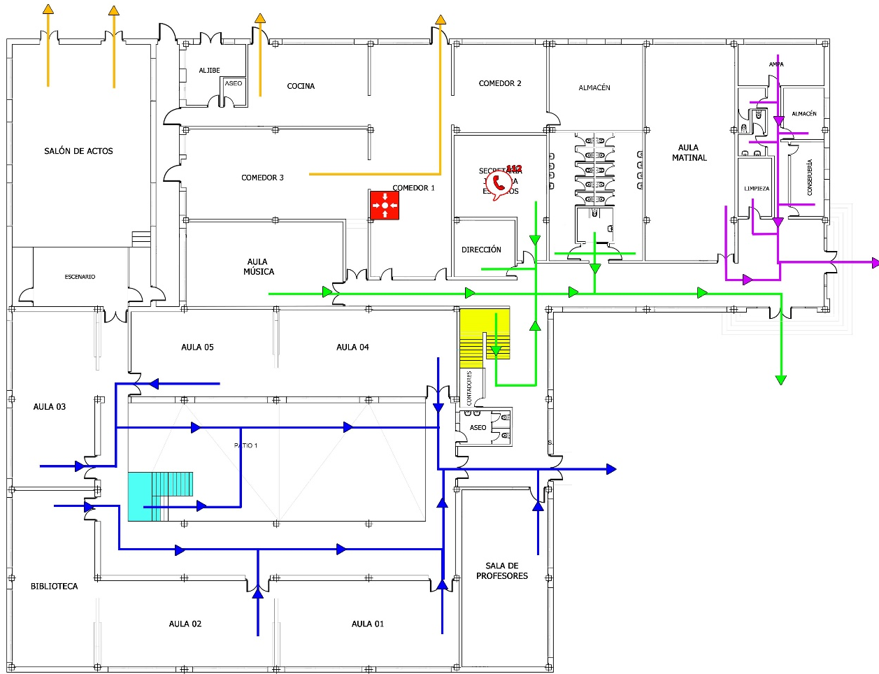
PLANTA BAJA
